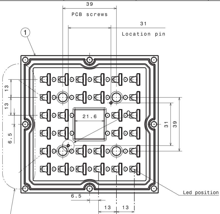
Detail C Scale: 2:1
